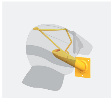
Helmdüsen
